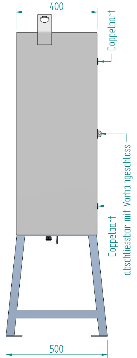
Schema Art.Nr. 231415
